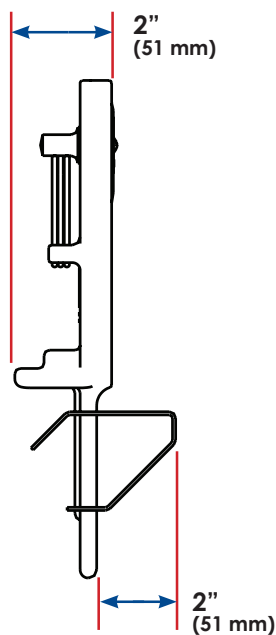
Suporte instalado para uso na altura da mesa de trabalho
