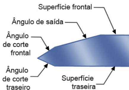
Perfil típico
